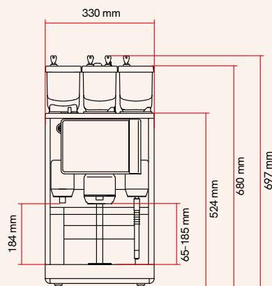
Schaerer Coffee Skye Frontansicht/ Seitenansicht rechts
